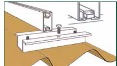
Montage der Tragschienen
