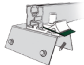
Fix2000 KlickTop
