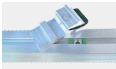
1 Kreuzverbinder am Unterprofil einhaken
