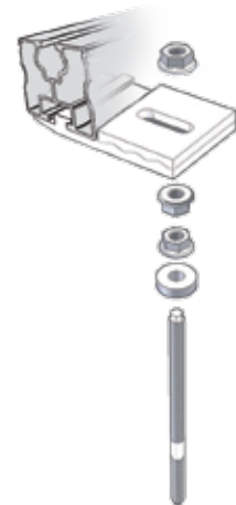
Welldachbefestigung KlickTop
